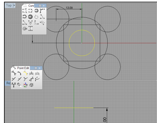
Рис.10. Положение окружностей малого радиуса
